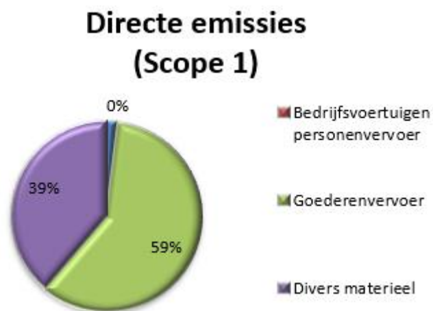
Figuur 2 – Overzicht verdeling emissies scope 1 in ton CO 2
